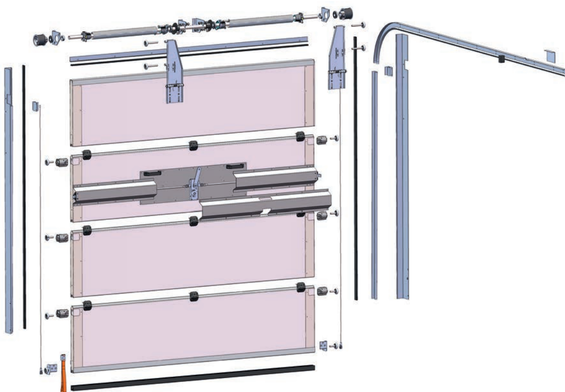
Principiální výkres vrat s vnitřním zajištěním
