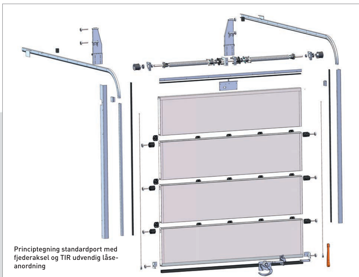
CARGO-ALUMINIUMPORT, sektionshøjder 250-300 mm
