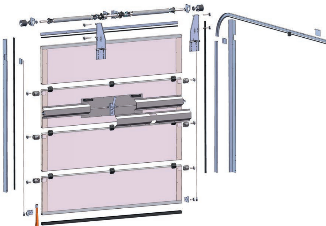
Belső zárszerkezetű hátfalak elvi rajza
