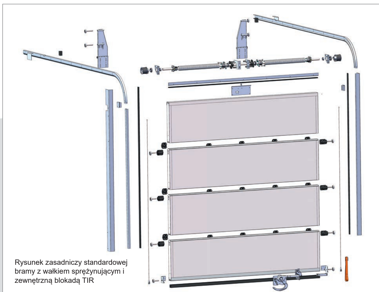
BRAMA ALUMINIOWA CARGO, wysokości sekcji 250-300 mm
