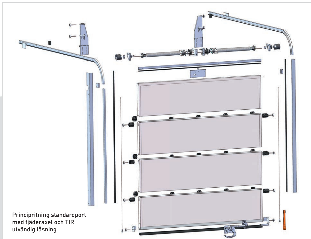
CARGO-ALUMINIUMPORT, sektionshöjder 250-300 mm
